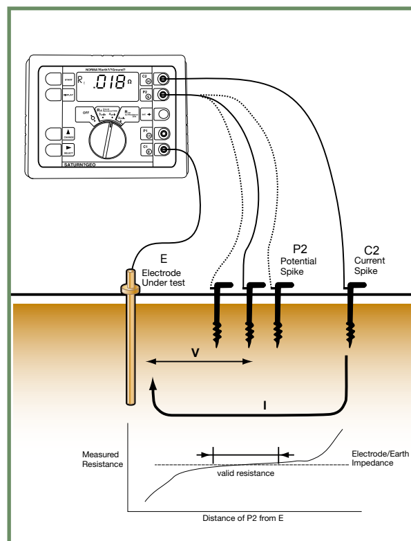
Figura 4. Esquema de conexión del telurómetro
