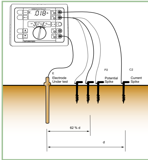
Figura 6: posiciones de las picas para la regla del 62%
