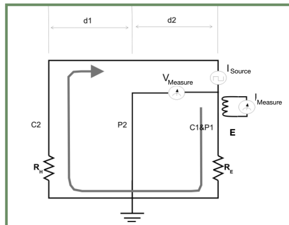
Figura 5. Circuito eléctrico de la medida
