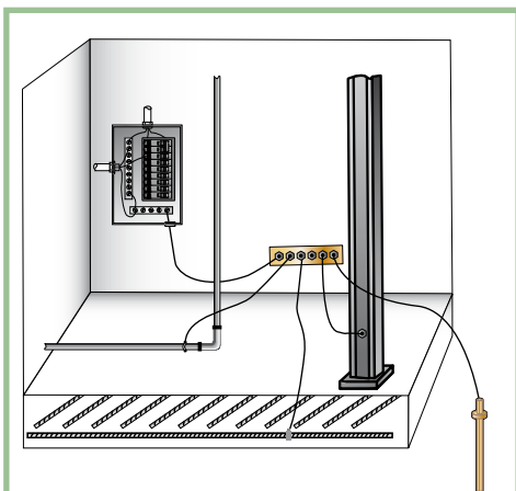
Figura 1. Instalación general de puesta a tierra
